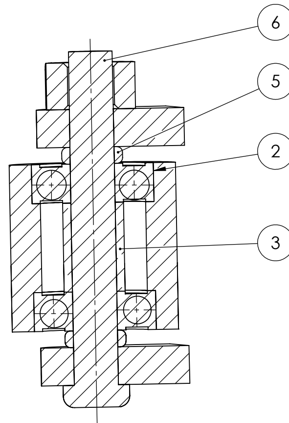
SECCIÓN B-B ESCALA 1.5 : 1
